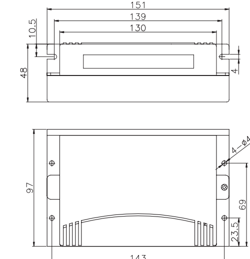
(d) Mechanical specifications of the EM806
